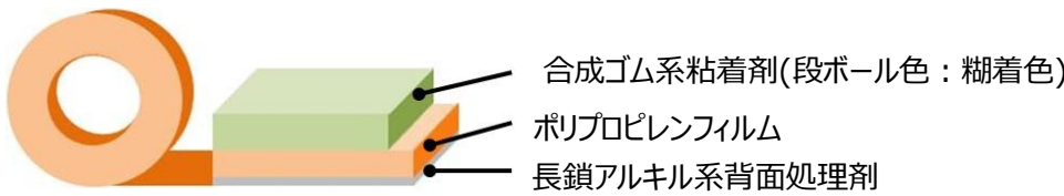
図 MR-3605 テープ構成
