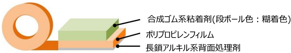
図 MR-3601 テープ構成
